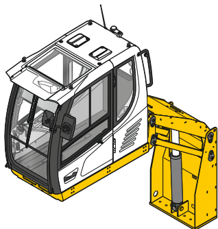
Hydraulische Kabinenerhöhung
